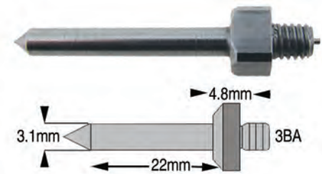
Long Case Clock - Rack Stud
